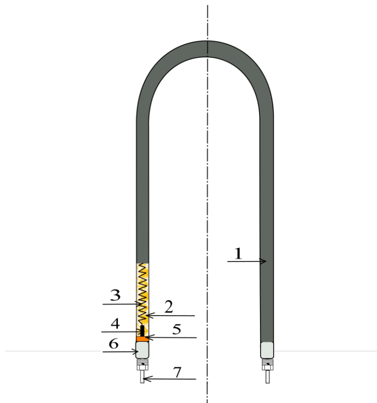
Типовые формы ТЭН
