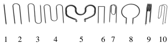
Типовые формы ТЭН
